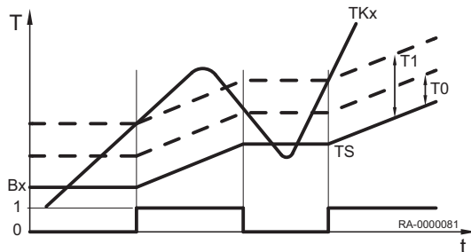
Obr.37 Naplňování zásobníku
