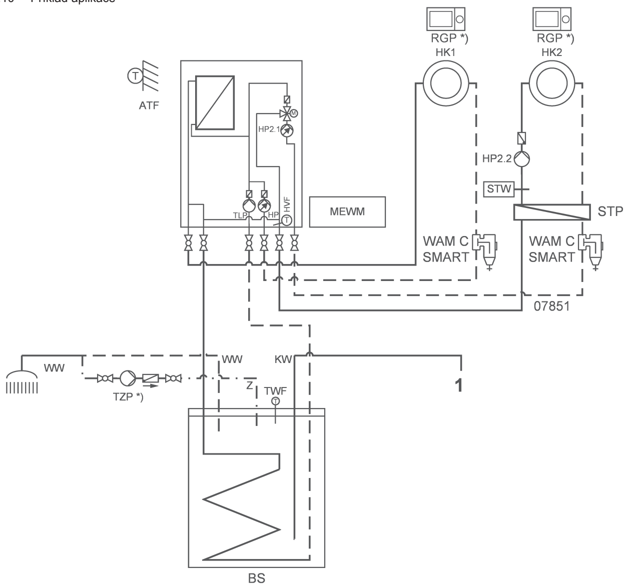
Obr.10 Příklad aplikace
