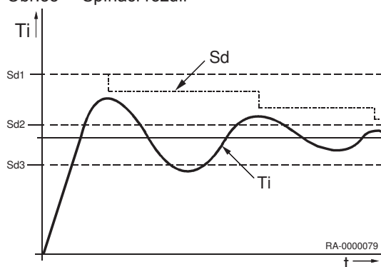
Obr.35 Spínací rozdíl
