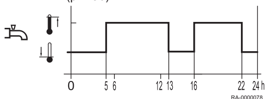
Obr.34 Spuštění dle časovacího programu 4 (příklad)
