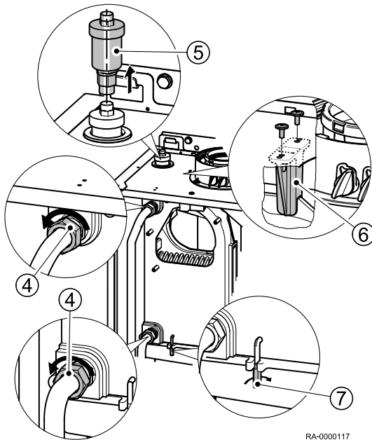
Obr.45 Demontáž tepelného výměníku
