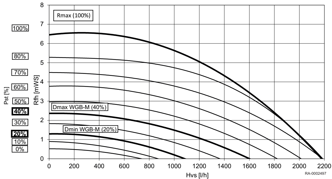
Obr.1 Celková čerpací výška WGB-M EVO pro čerpadlo topného okruhu
