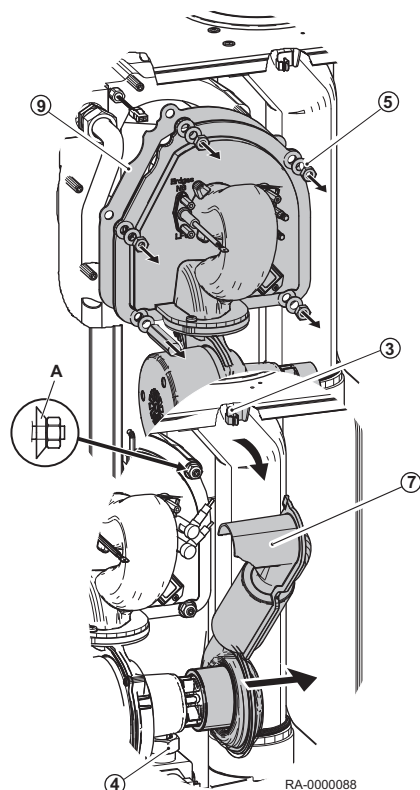
Obr.44 Demontáž hořáku
