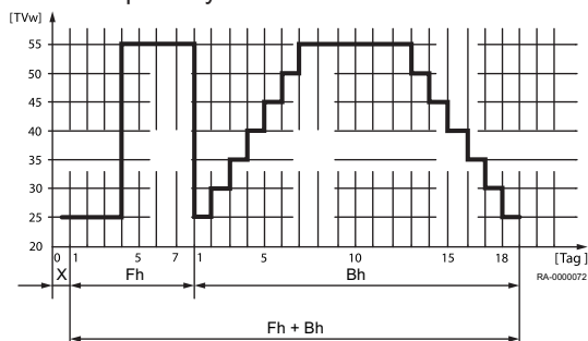
Obr.32 Profil teplot funkce vytápění podlahy
