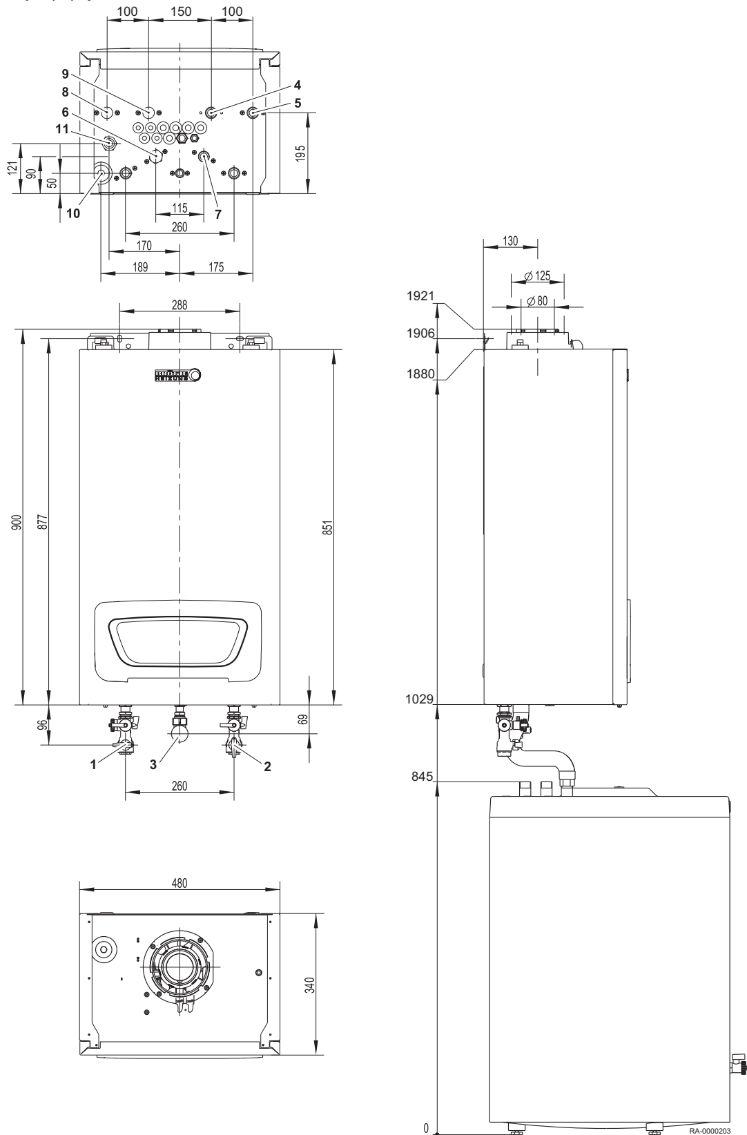
Obr.3 Rozměry a připojení WGB-M EVO
