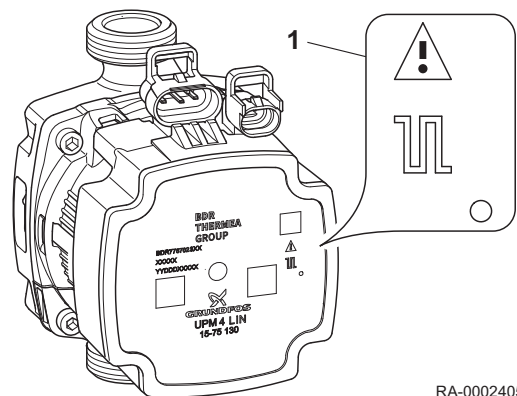
Obr.22 Stavový displej Čerpadlo topného okruhu UPM4
