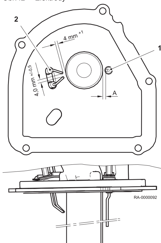
Obr.42 Elektrody
