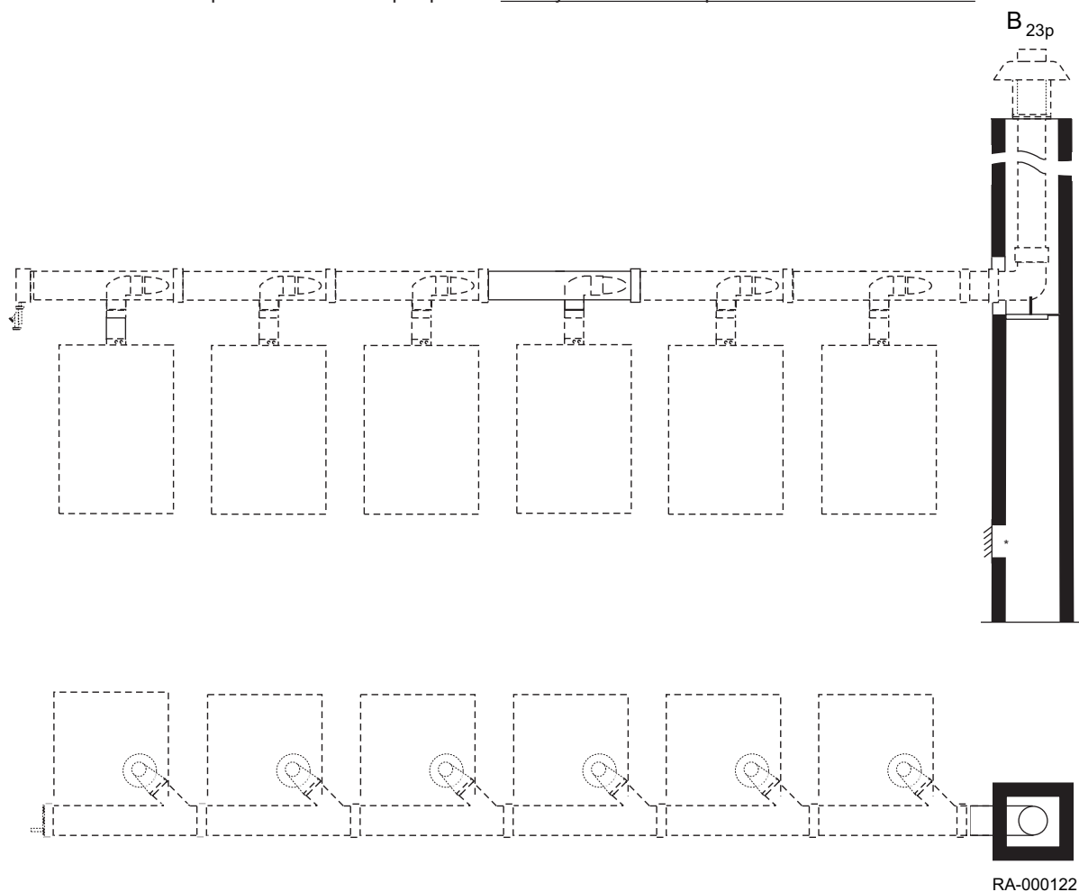
Obr.16 Soustava spalinového vedení pro provoz závislý na vzduchu z prostoru instalovaného kotle
