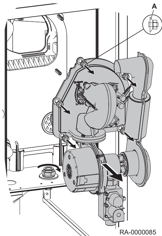
Obr.40 Demontáž hořáku
