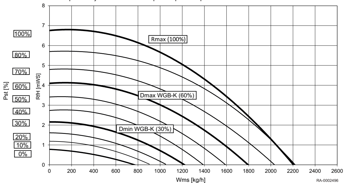
Obr.1 Celková dopravní výška WGB-K EVO pro čerpadlo topného okruhu
