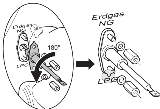
Obr.20 Změna na LPG
