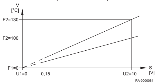
Obr.36 Příklad požadavku na teplo 10 V
