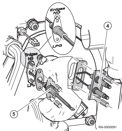
Obr.39 Demontáž zapalovací elektrody a ionizační sondy
