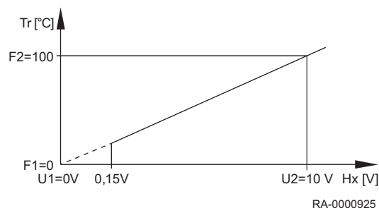
Obr.34 Hodnota napětí/hodnota funkce
