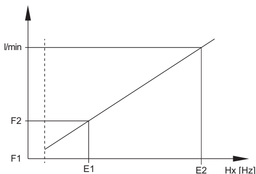
Obr.35 Příklad dvou různých křivek čidel
