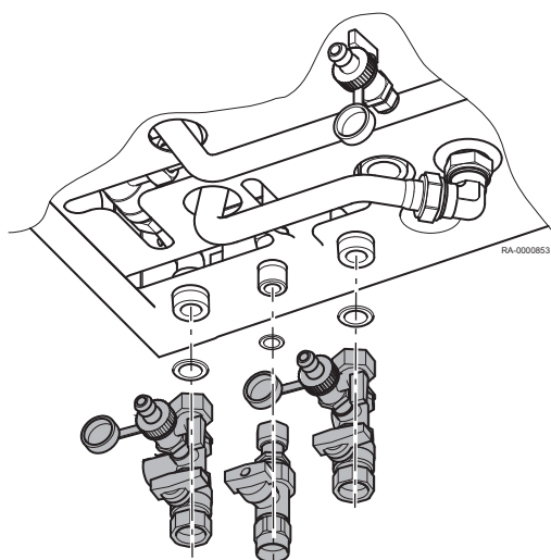
Obr.11 Instalace uzavíracích kohoutů
