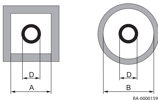
Obr.17 Minimální rozměry kouřovodu
