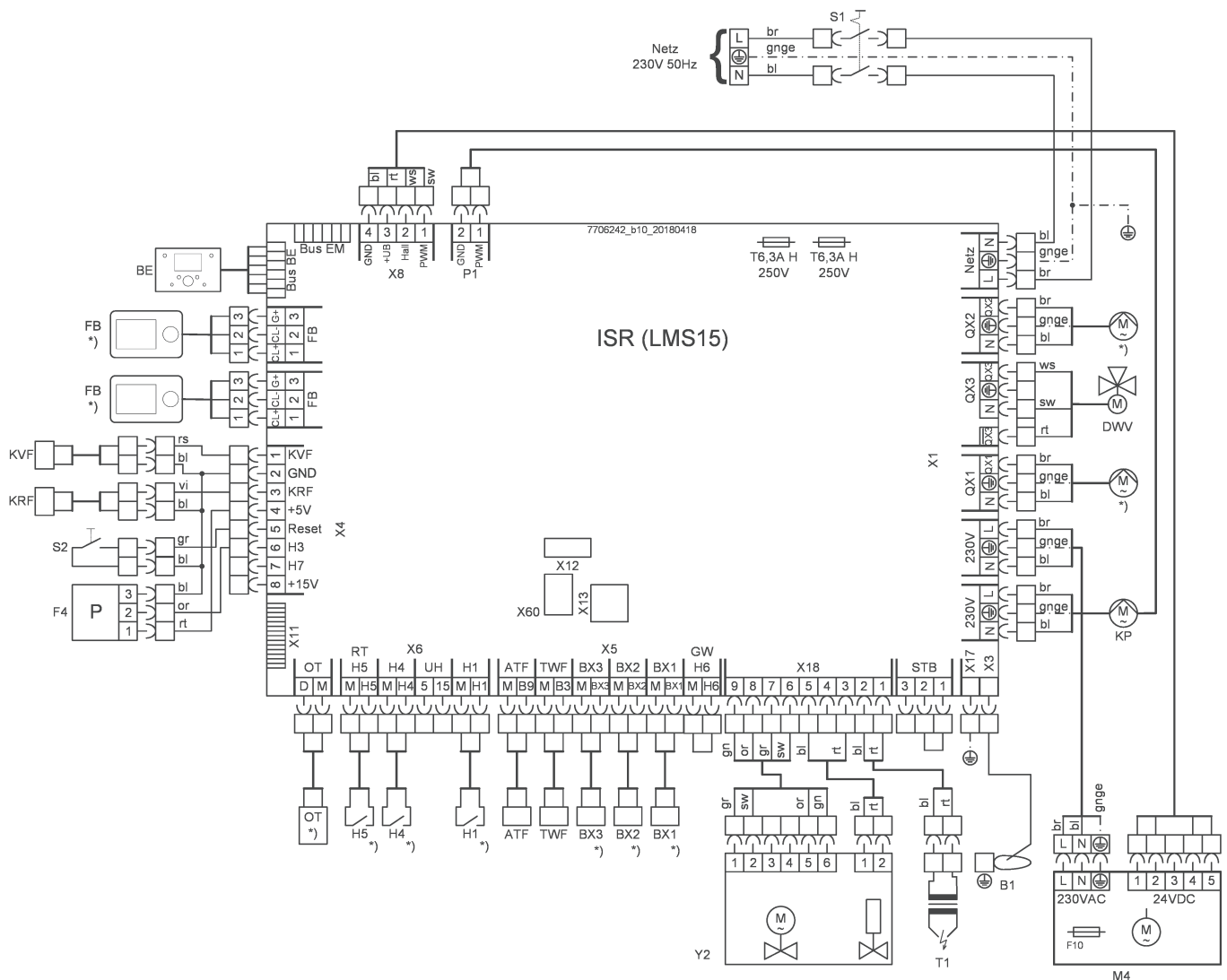
Obr.3 Schéma zapojení WGB-K EVO
