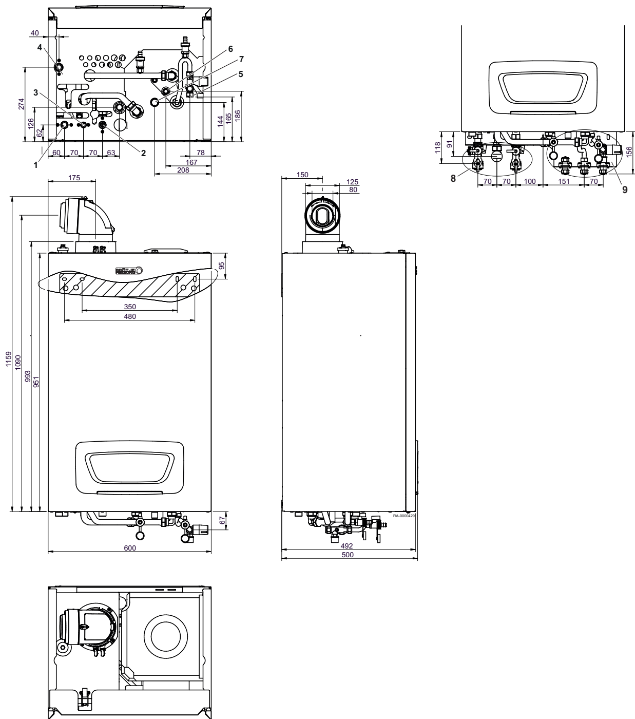
Obr.2 Rozměry a připojení WGB-K EVO
