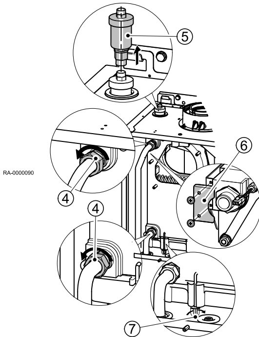
Obr.41 Demontáž tepelného výměníku
