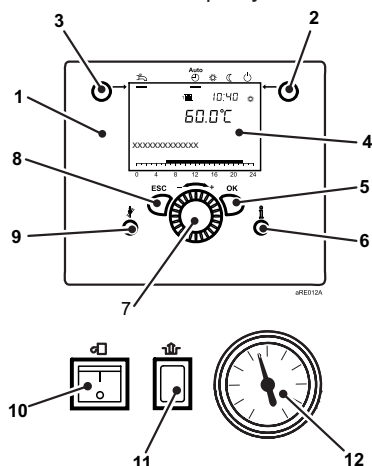
Obr.5 Provozní prvky
