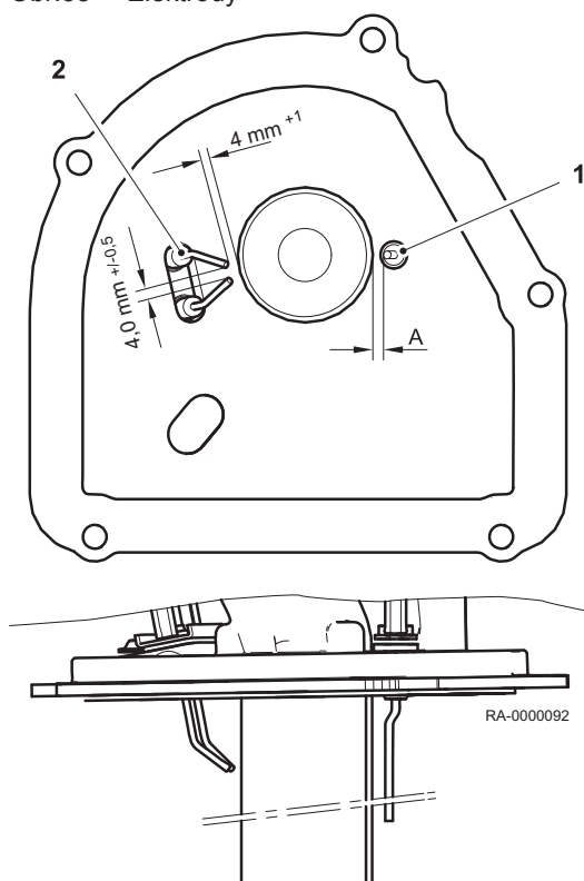
Obr.38 Elektrody
