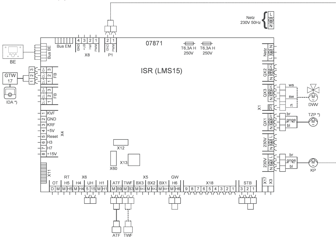
Obr.10 Schéma zapojení
