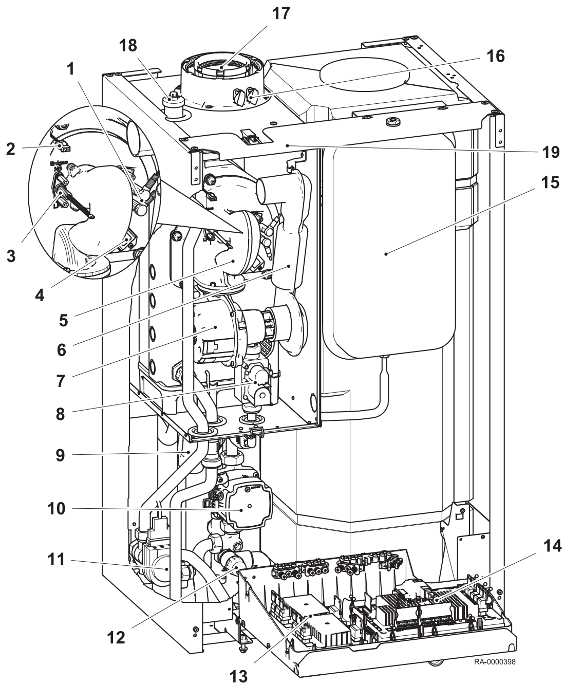
Obr.4 Náhled na kotel WGB-K EVO (zobrazení bez přední stěny a krytu regulační jednotky)
