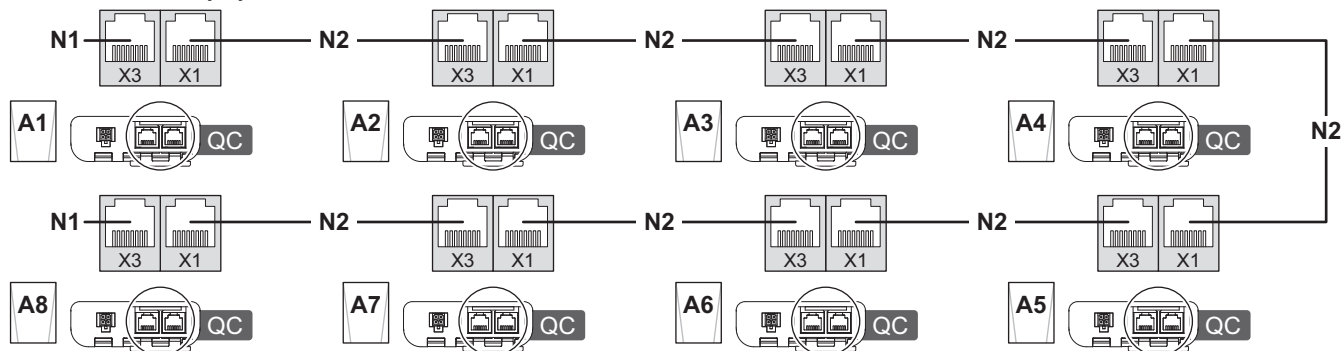
Obr.49 Kaskádový systém
