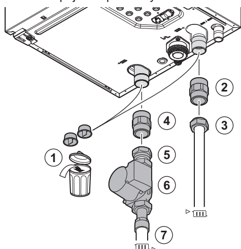
Obr.39 Připojení topného systému
