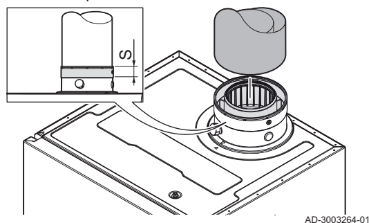
Obr.42 Připojení přívodu vzduchu a odvodu spalin
