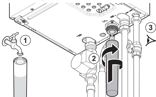
Obr.101 Napuštění sifonu
