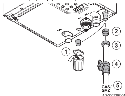
Obr.41 Připojení plynového potrubí
