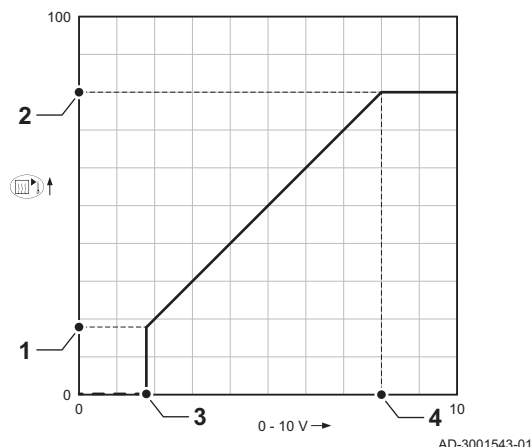
Obr.88 0–10V řízení
