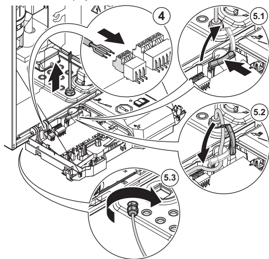
Obr.54 Připojení kabelu
