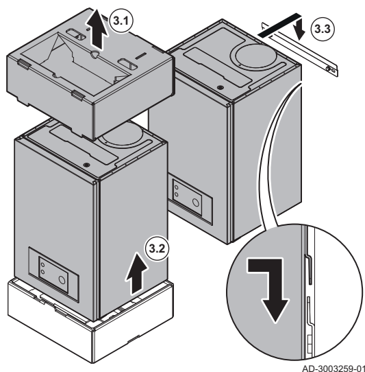
Obr.37 Umístění kotle
