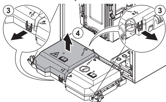
Obr.52 Zvedněte kryt
