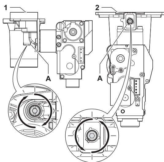
Obr.106 Poloha seřizovacího šroubu A
