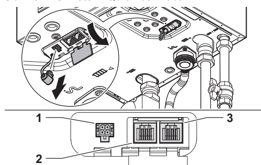
Obr.46 Umístění Quick connect
