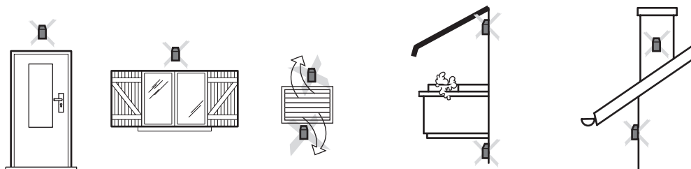
Obr.45 Montáž čidla venkovní teploty
