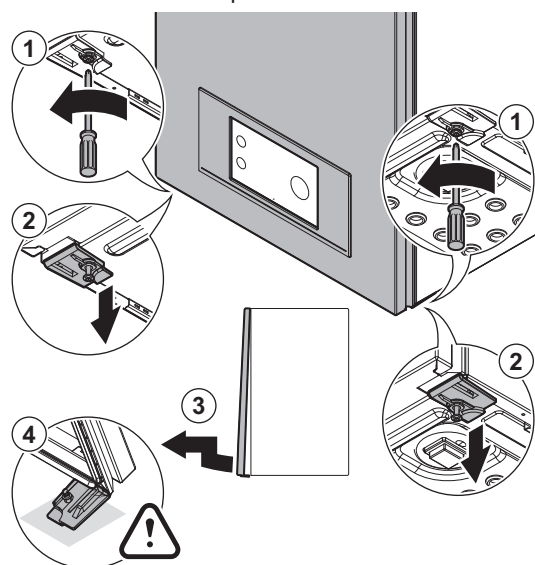
Obr.123 Demontáž panelu
