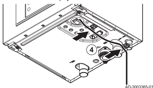
Obr.38 Vedení napájecího kabelu
