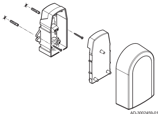
Obr.45 Montáž čidla venkovní teploty
