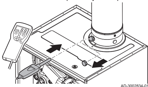
Obr.107 Vložte sondu pro analyzátor spalín
