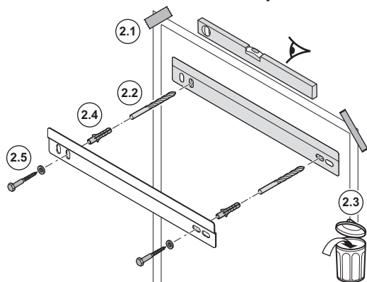
Obr.36 Instalace nástěnné konzoly
