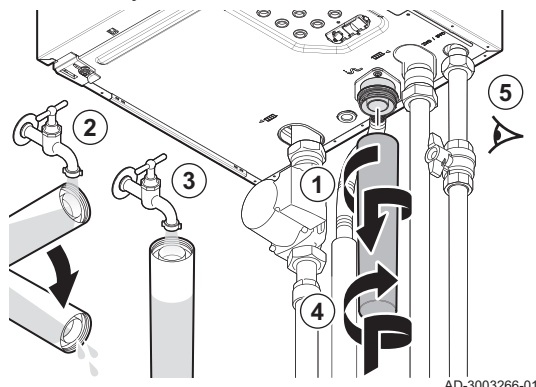
Obr.124 Vyčištění sifonu
