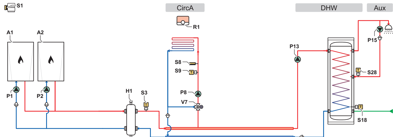
Obr.23 Schéma a součásti - 6000143
