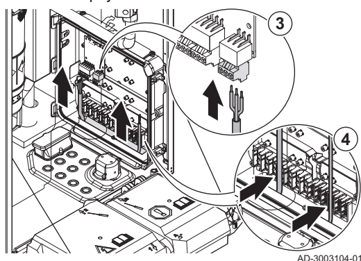
Obr.57 Připojení kabelu
