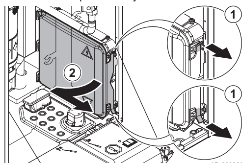
Obr.55 Přístup k rozšiřujícímu modulu
