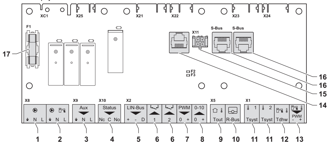
Obr.58 Propojovací elektronická deska CB-25
