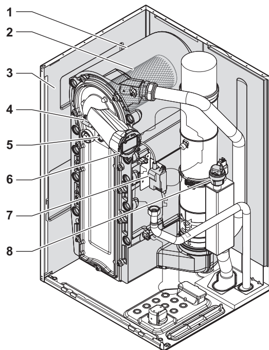
Obr.2 Vnitřní
