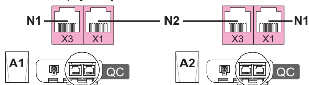
Obr.30 Připojení systémové sběrnice - Hlavní kotel A1 do Podružný kotel A2
