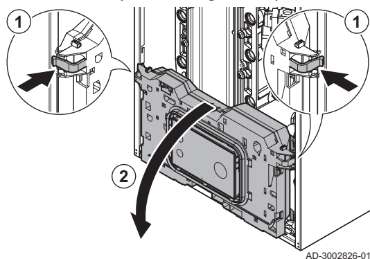
Obr.52 Zvedněte kryt
