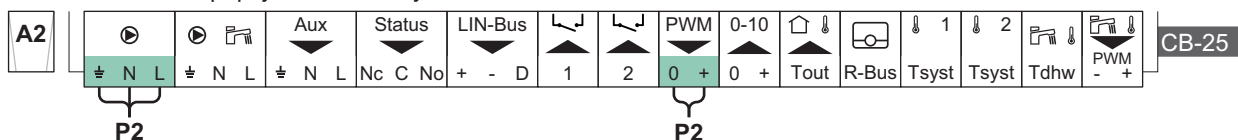
Obr.25 Elektrické připojení - Podružný kotel A2
