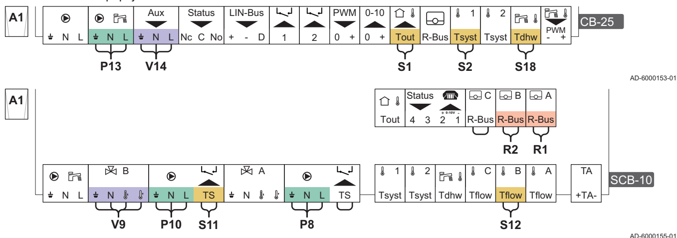
Obr.32 Elektrické připojení - Hlavní kotel A1
