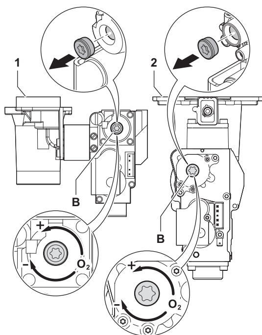
Obr.111 Poloha seřizovacího šroubu B
