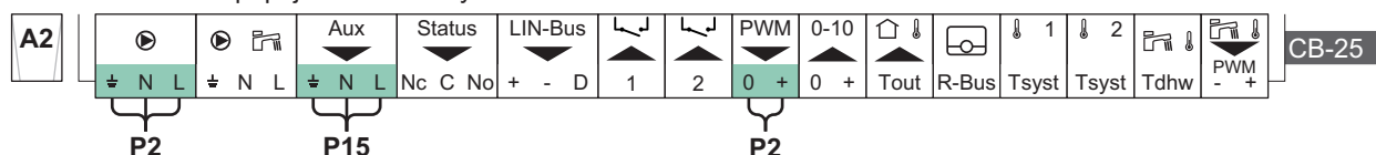
Obr.29 Elektrické připojení - Podružný kotel A2
