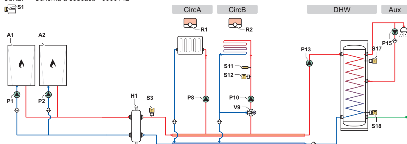
Obr.27 Schéma a součásti - 6000142
