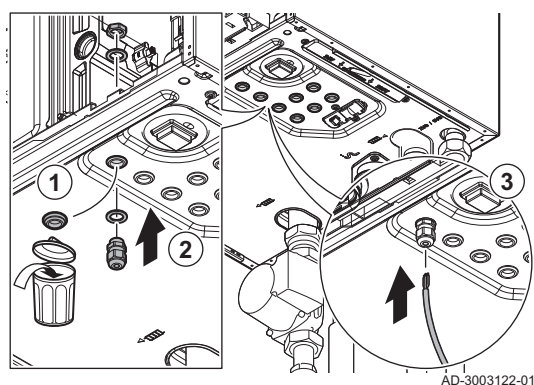
Obr.53 Vedení kabelů
