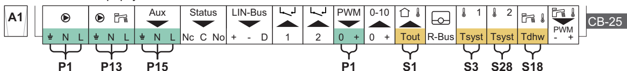
Obr.24 Elektrické připojení - Hlavní kotel A1
