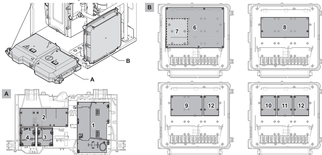
Obr.50 Umístění elektronických desek
