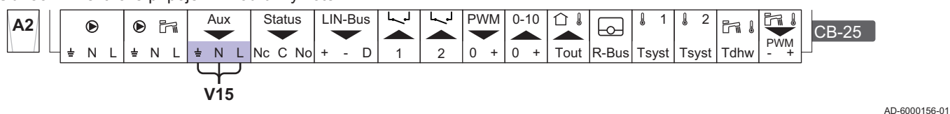
Obr.33 Elektrické připojení - Podružný kotel A2
