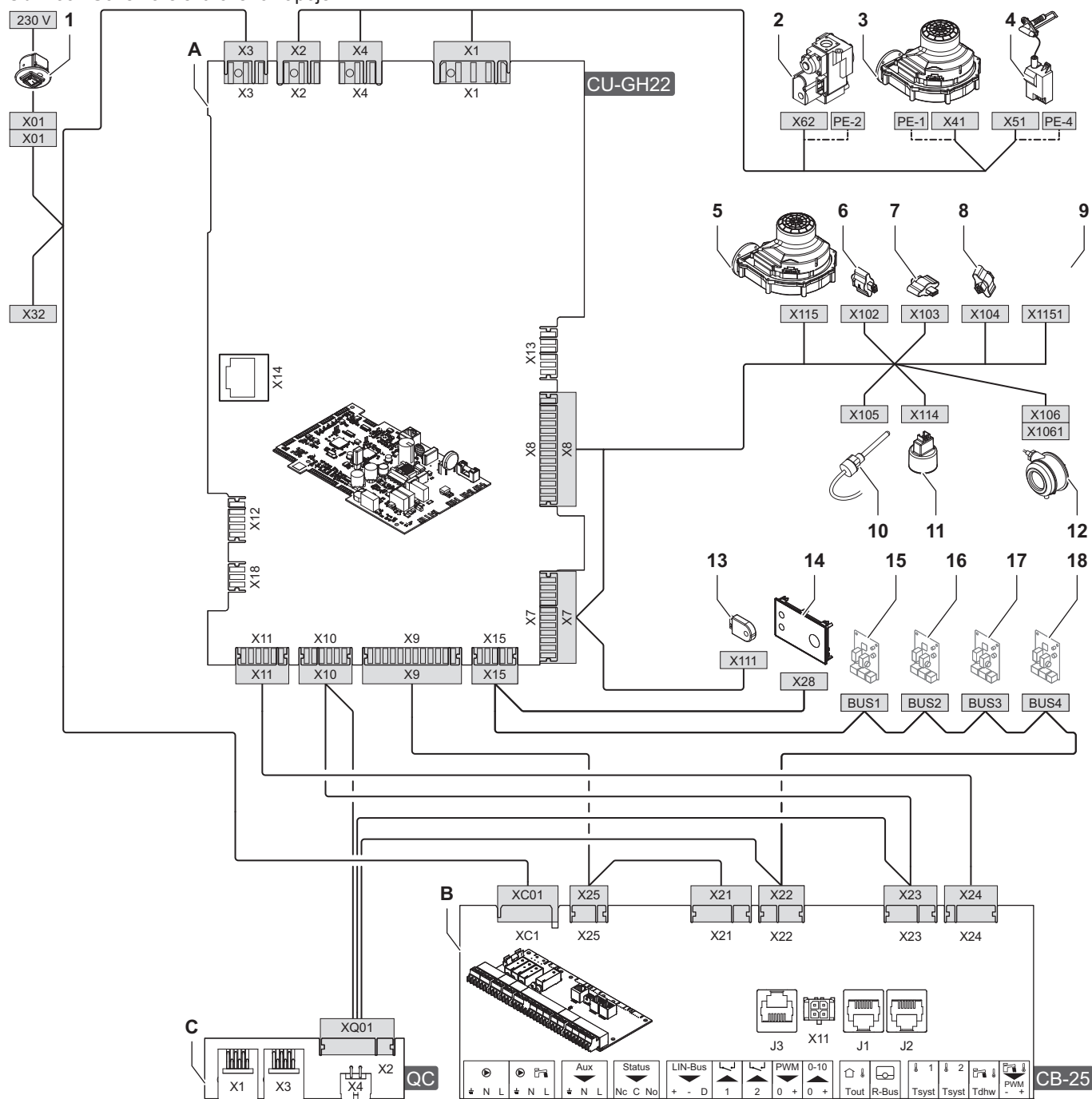
Obr.139 Schéma elektrického zapojení
