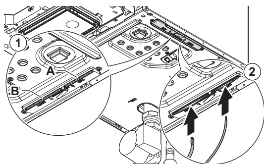
Obr.56 Vedení kabelů
