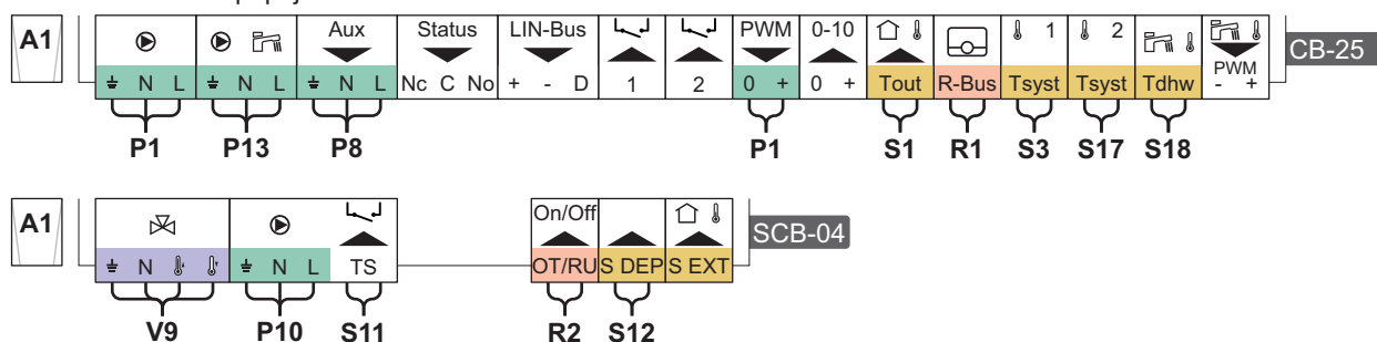
Obr.28 Elektrické připojení - Kotel A1
