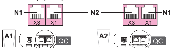
Obr.26 Připojení systémové sběrnice - Hlavní kotel A1 do Podružný kotel A2
