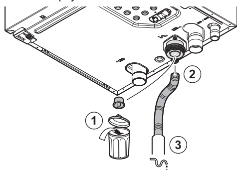
Obr.40 Připojení odvodu
