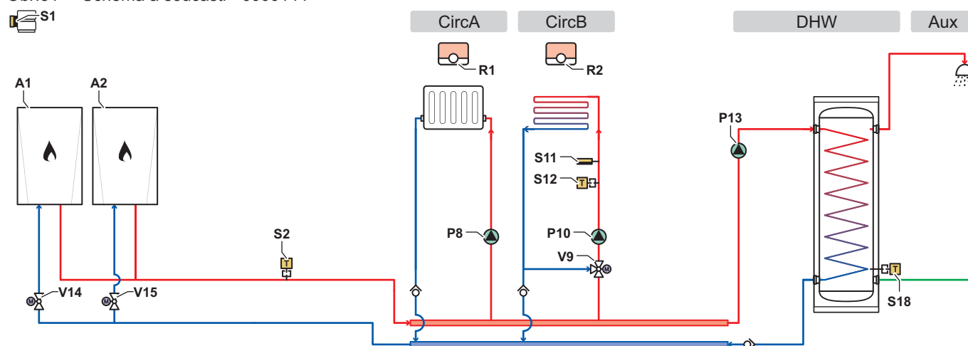
Obr.31 Schéma a součásti - 6000144
