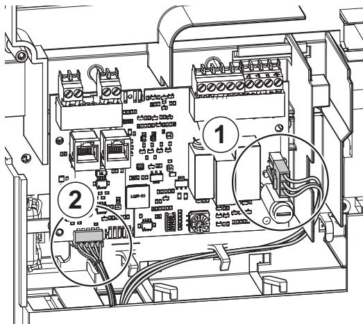
Obr.4 Elektrické připojení rozšiřovacího modulu SCB-04
