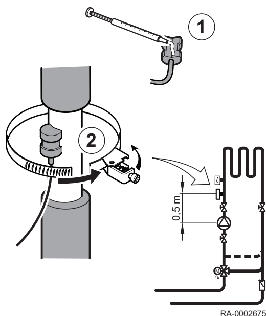
Obr.10 Montáž čidla výstupní teploty
