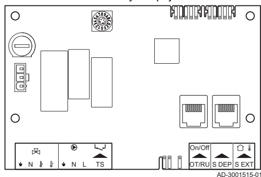
Obr.2 Deska s tištěnými spoji SCB-04
