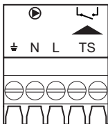
Obr.6 Konektor čerpadla a ochranného termostatu
