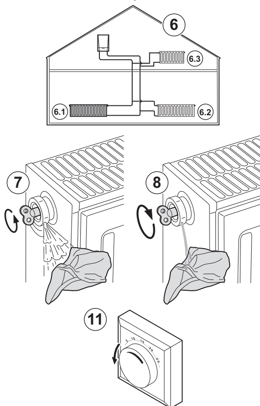
Obr.22 Odvzdušnění systému
