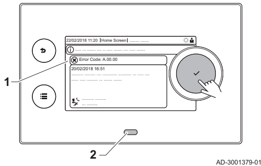
Obr.23 Zobrazení chybového kódu na IWR Alpha
