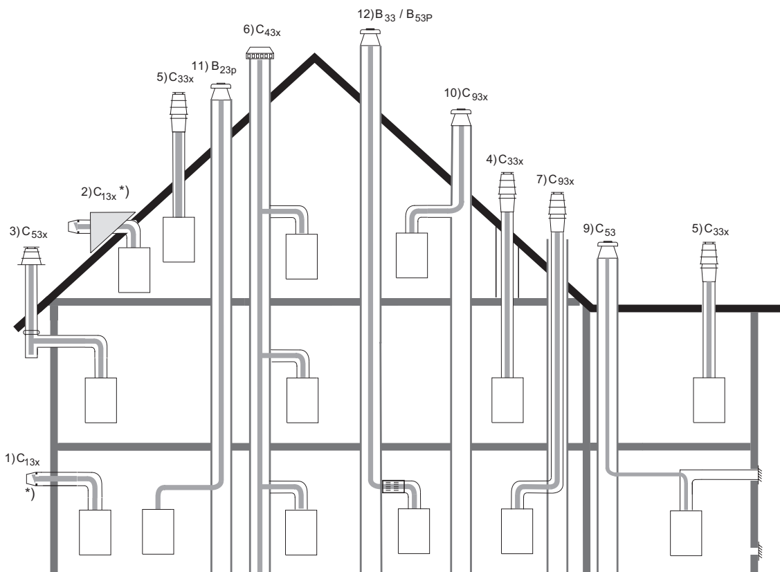
Obr.13 Možnosti připojení se systémem KAS (příslušenství)
