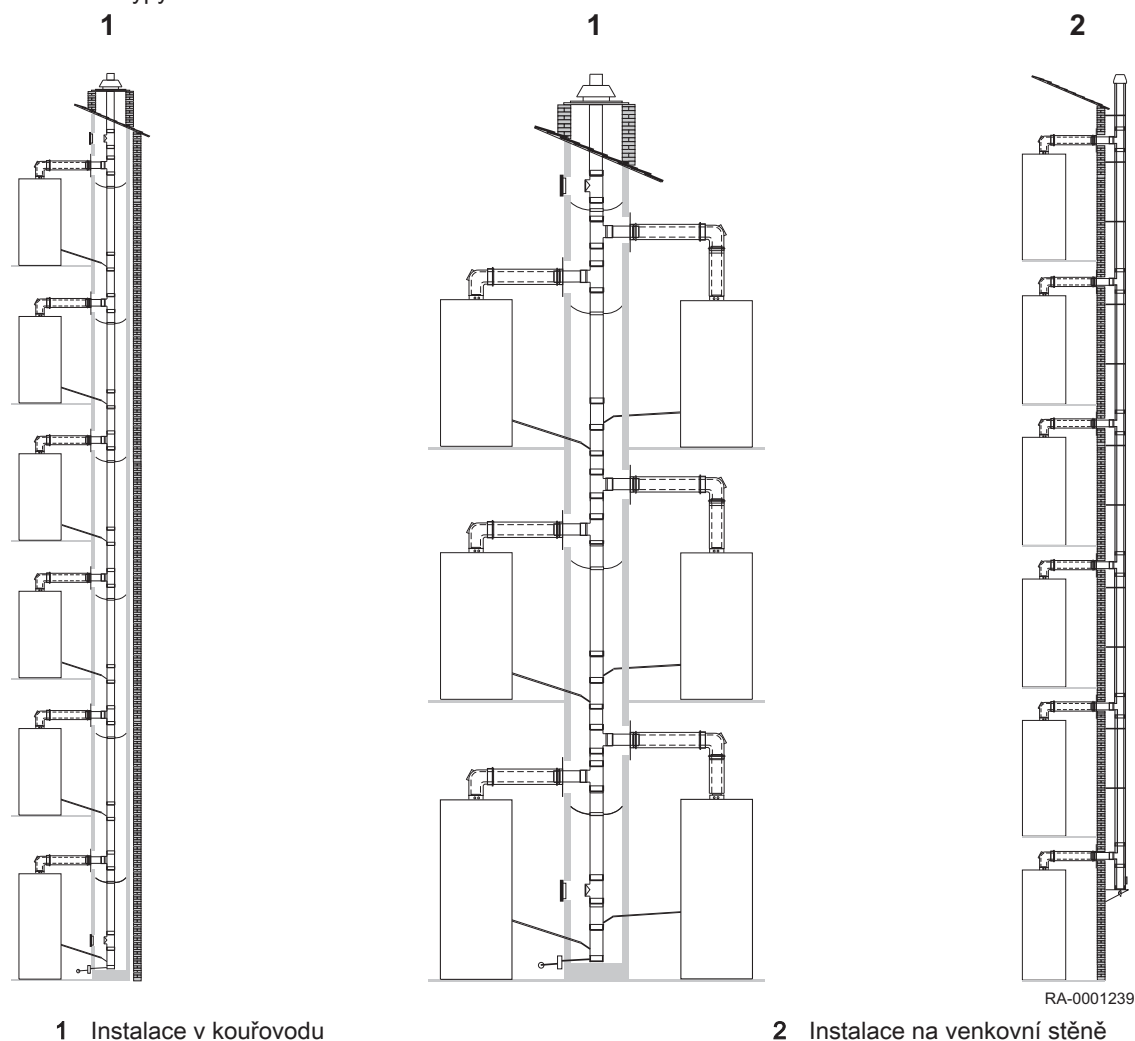
Obr.19 Typy soustav
