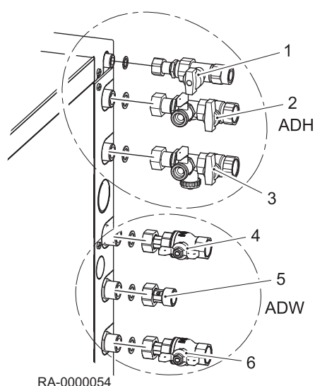
Obr.11 Instalace uzavíracích kohoutů
