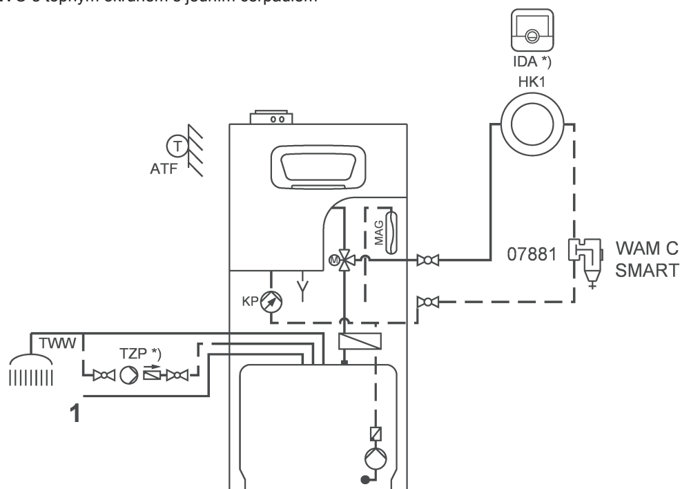
Obr.9 BBK EVO s topným okruhem s jedním čerpadlem
