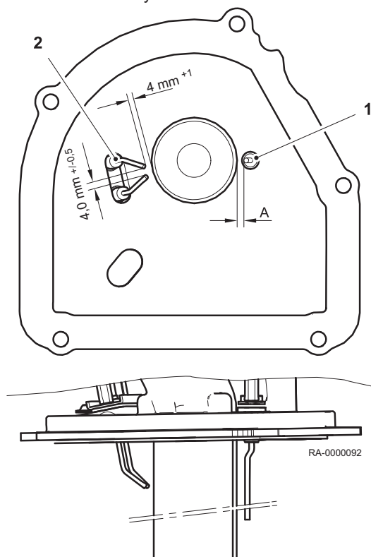
Obr.38 Elektrody
