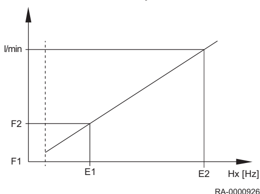
Obr.36 Příklad dvou různých křivek čidel
