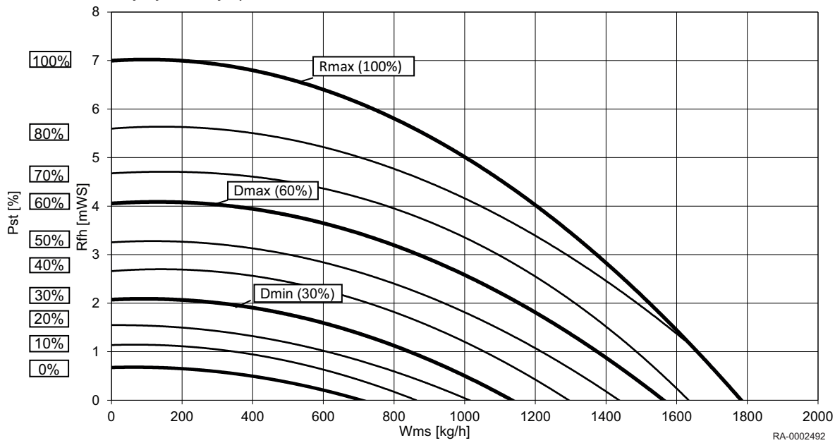
Obr.1 Celkový dynamický spád BBK EVO 20/22
