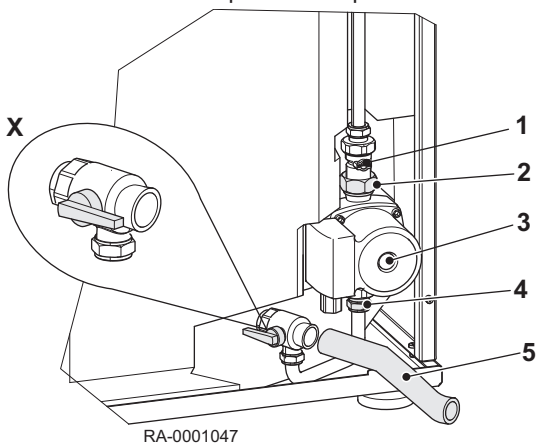
Obr.42 Demontáž plnicího čerpadla TUV
