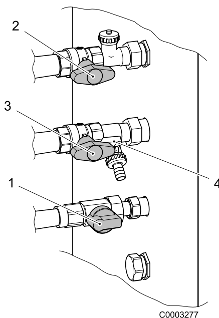
Obr. 5: Zavřete uzavírací ventily a uzavírací ventil plynu
