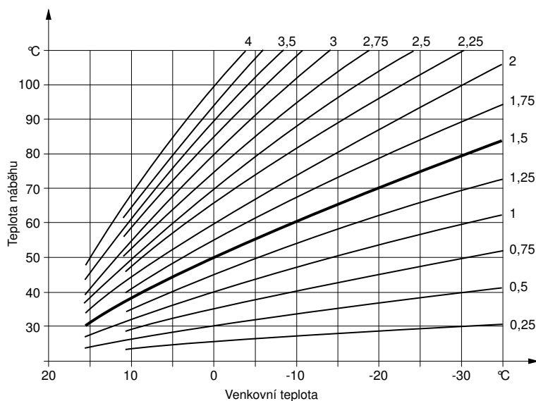
Obr. 4: Topná křivka
