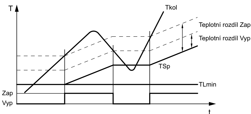
Obr. 29: Laderegelung /schematisch)
