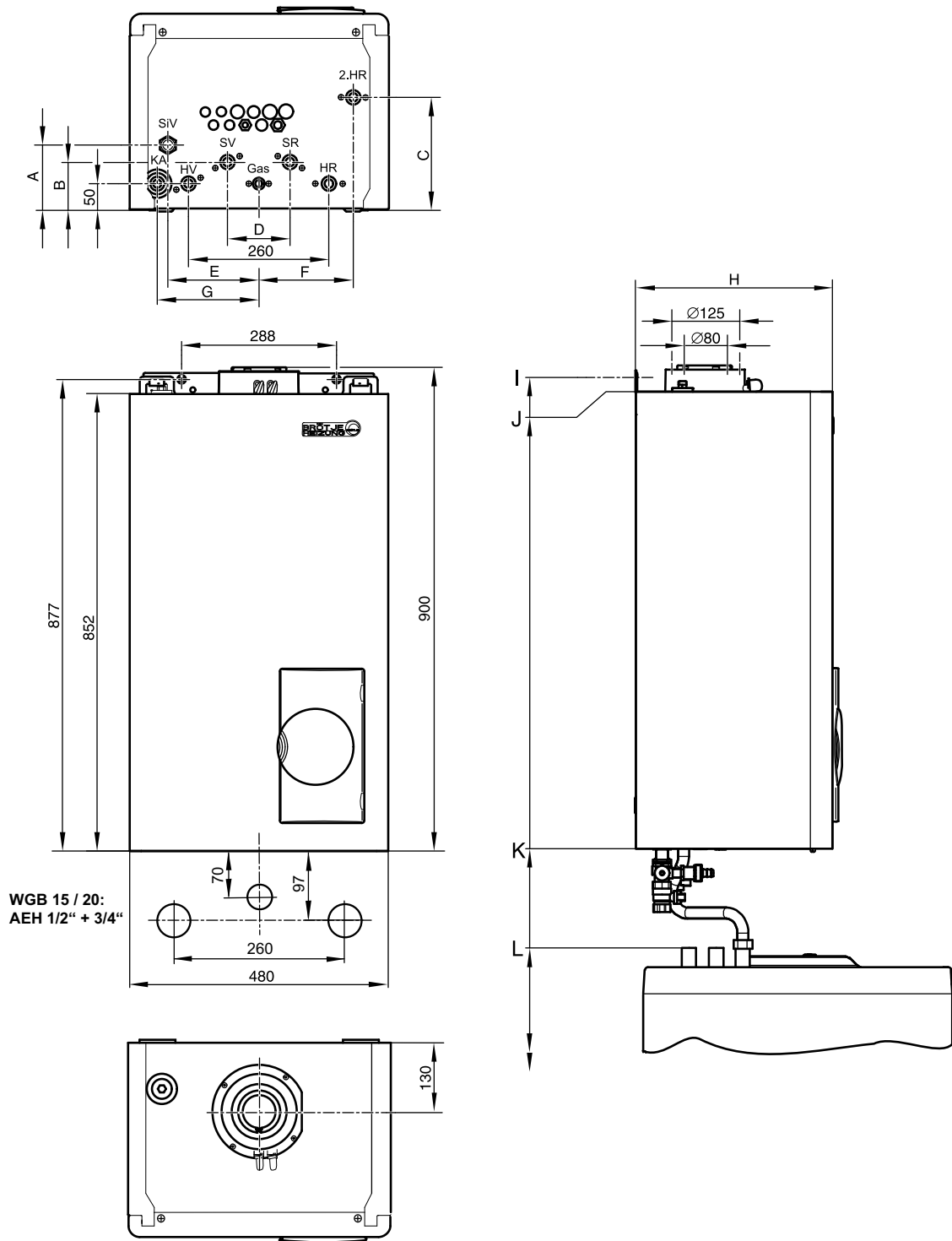
Obr. 1: Rozměry a přípojky kotle
