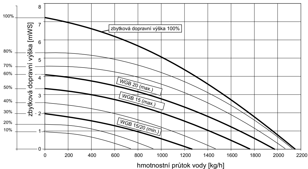
Obr. 25: Zbytková dopravní výška WGB 15-38 E
