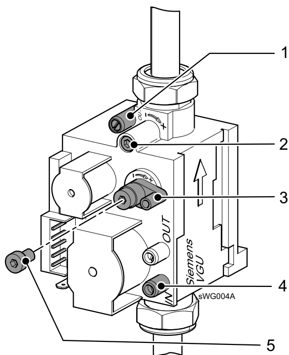
Obr. 14: Plynová armatura (nastavení tlaku v trysce šroubovacím nástavcem Torx T15)
