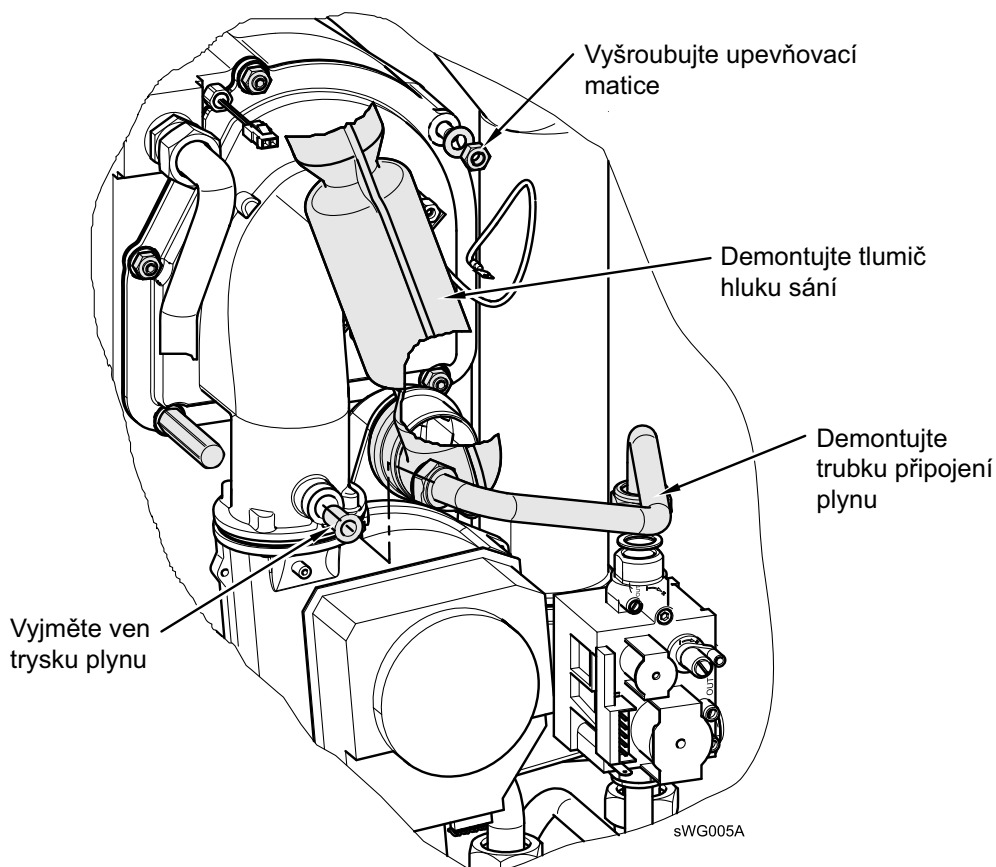
Obr. 35: Demontáž plynového hořáku
