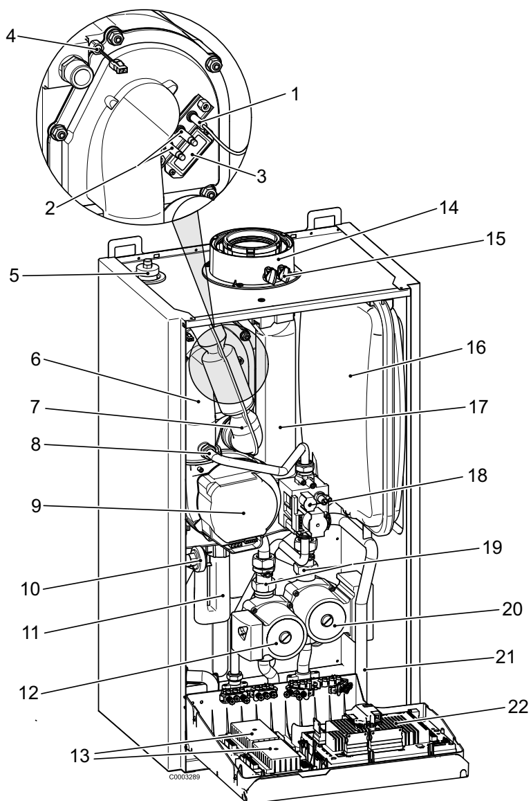
Obr. 36: Zobrazení kotle WGB (bez přední stěny a krytu regulace)
