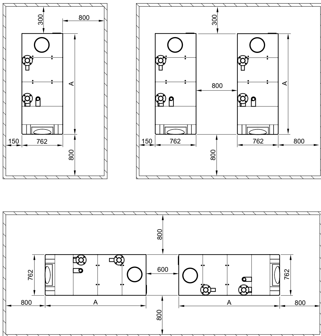
Abb 32: Empfohlener Platzbedarf
