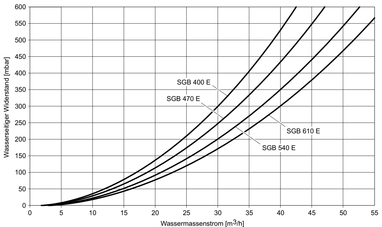
Abb 10: Diagramm Wasserseitiger Widerstand SGB 400 - 610 E
