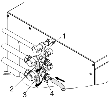
Obr. 5: Zavřete uzavírací ventily a uzavírací ventil plynu
