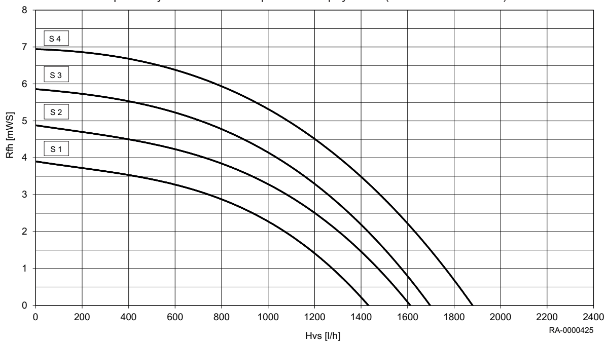
Obr.2 Celková dopravní výška WGB-M EVO pro míšící topný okruh (úroveň nastavení 1-4)
