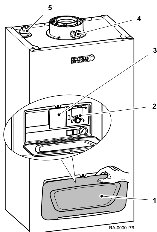
Obr.1 Přehledový diagram WGB EVO
